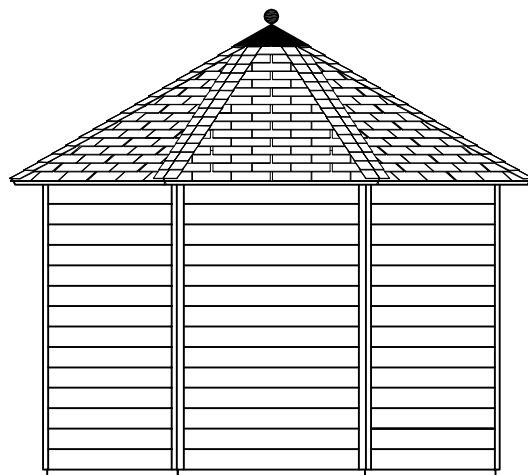
Achteraanzicht / Rear view / Hinterseite
