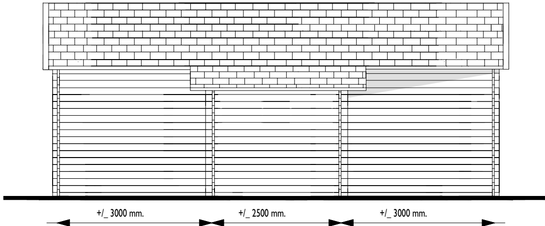
Achter aanzicht Hinten Ansicht Rear view
